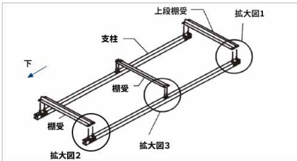
●拡大図1：支柱に上下棚受をつけます
